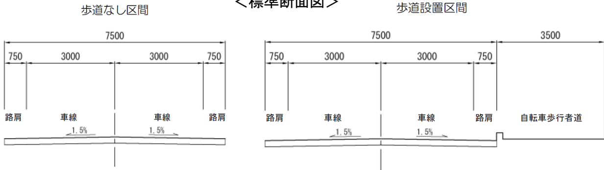
＜標準断面図＞
